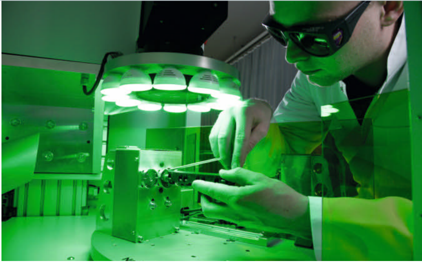
Bild 1. Laserdirektstrukturierung mit mehreren Lasern (Foto:LPKF)
